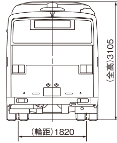
■前乗 ホイールベース:6,000mm
