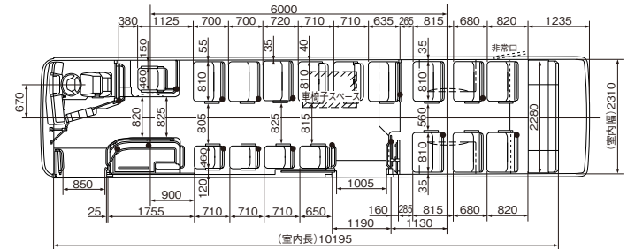
■郊外II型 中乗 ホイールベース:6,000mm
