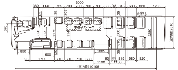
■ラッシュ型 中乗 ホイールベース:6,000mm
