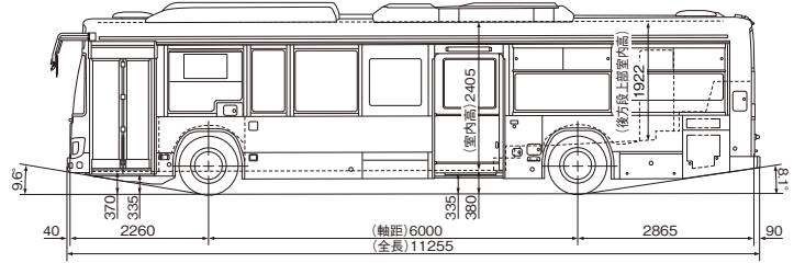
■中乗 ホイールベース:6,000mm
