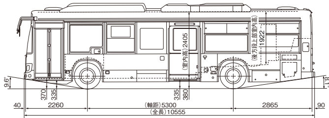
■中乗 ホイールベース:5,300mm
