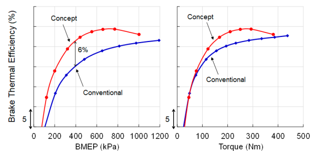
図6 正味熱効率のシミュレーション結果
