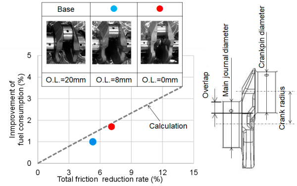
図14 クランク摩擦力の低減効果
