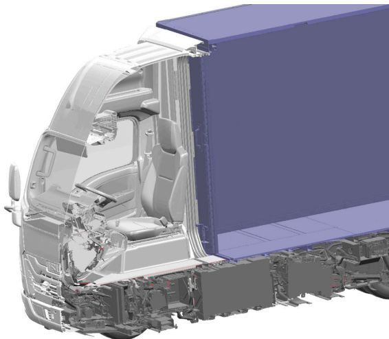
図3 シャシ概要
