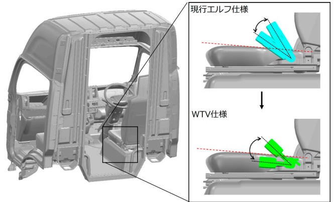
図12 運手席シートベルトバックル回転
