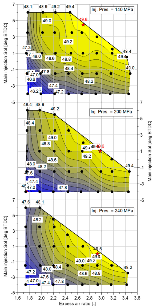
図5 燃料噴射量 117\text{mm}^3/\text{cycle} 、燃焼噴射圧力140MPa(上図)、200MPa(中図)、240MPa(下図)の条件での図示熱効率コンター図
