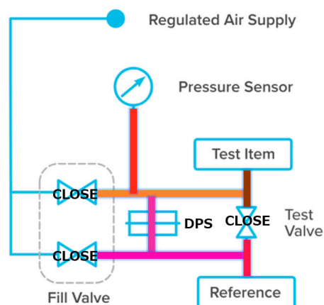
図6 リークテスト検査時状態図
