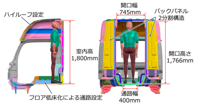
図4 主要寸法
