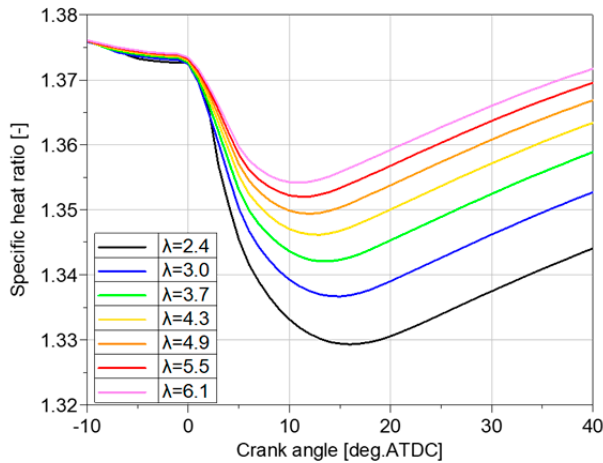
図9 HIDECSを用いた計算における空気過剰率の違いによる比熱比の履歴の比較
