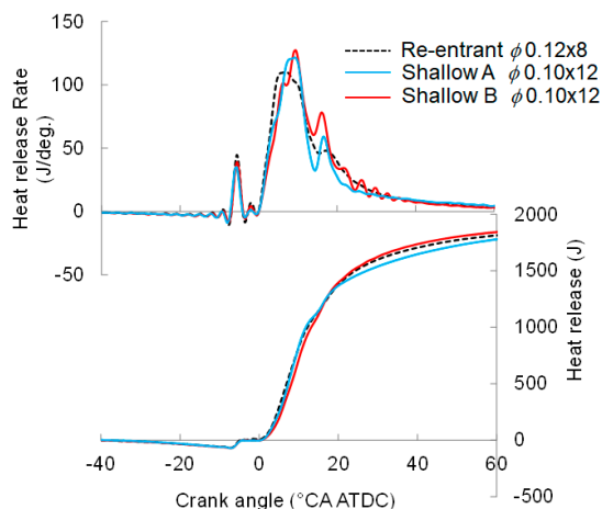
図9 条件2の熱発生率の比較
