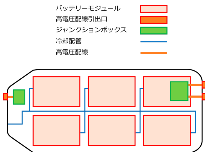
図2 バッテリーモジュール/冷却システム
