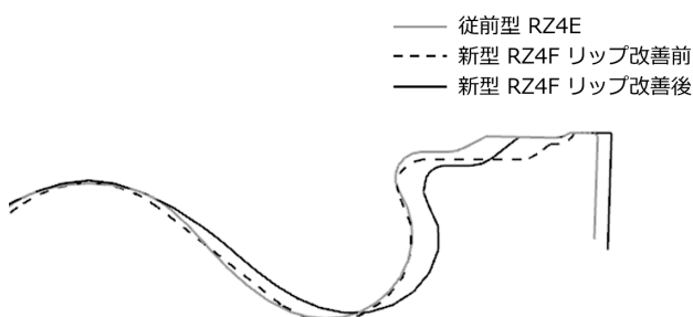
図10 ピストン燃焼室形状
