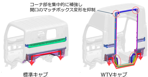
図5 ボディ背面のロードパス比較
