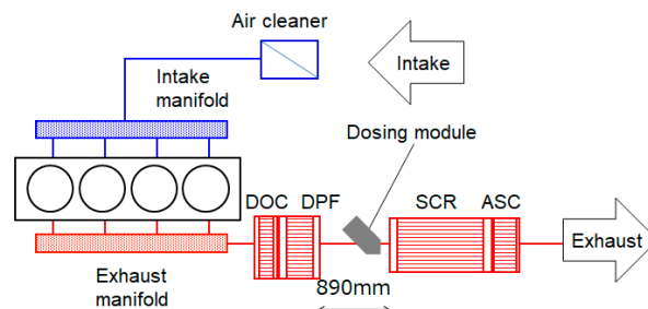
図10 エンジンシステム構成図
