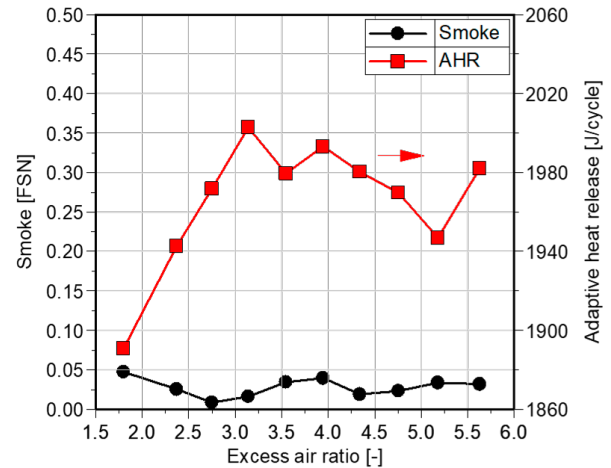
図3 燃料噴射量 66\text{mm}^3/\text{cycle} 、燃焼噴射圧力200MPa、メイン噴射開始時期1.0deg.BTDCの条件でのスモーク排出量と総発生熱量の比較
