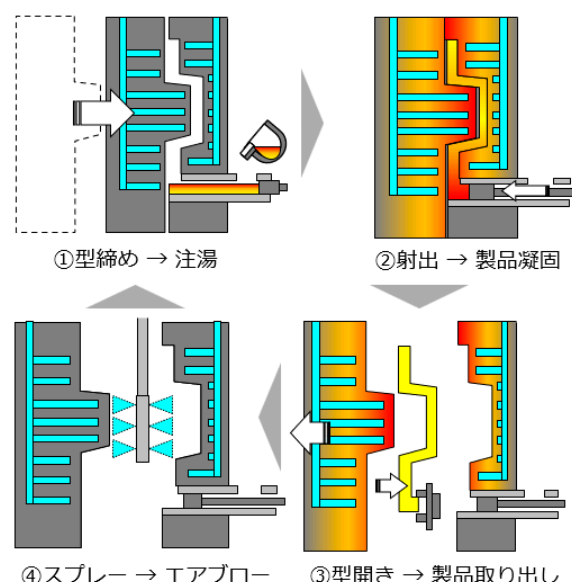
図1 ダイカスト工程フロー
