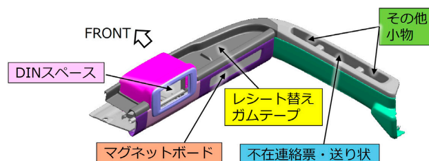
図9 ヘッダートレイ収納部
