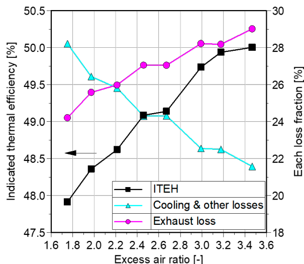
図7 燃料噴射量 117\text{mm}^3/\text{cycle} 、燃料噴射圧力 200\text{MPa} 、メイン噴射開始時期 1.0\text{deg.BTDC} の条件での図示熱効率、排気損失及び冷却その他損失割合の比較
