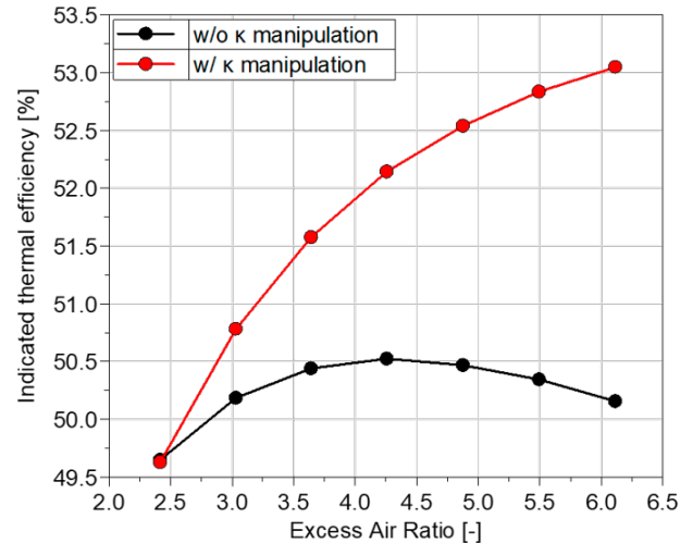
図11 HIDECSを用いた計算での膨張行程の比熱比の違いによる図示熱効率の比較
