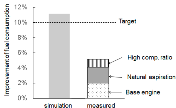
図14 重量車燃費の改善効果
