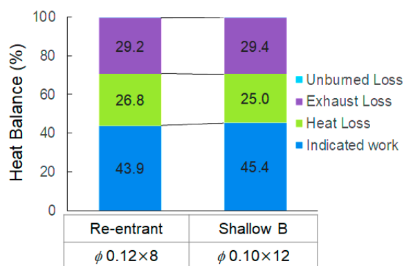
図10 条件2のヒートバランスの比較
