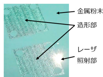
図8 PBF方式による造形の様子
