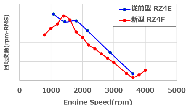
図16 エンジン回転変動
