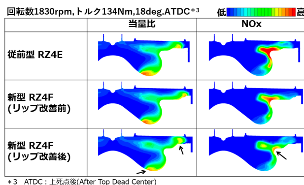
図11 燃焼解析結果
