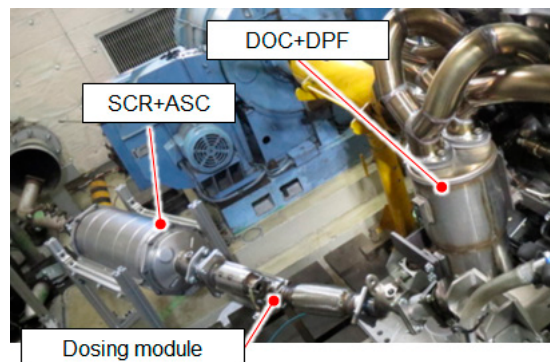
図11 評価用後処理システム
