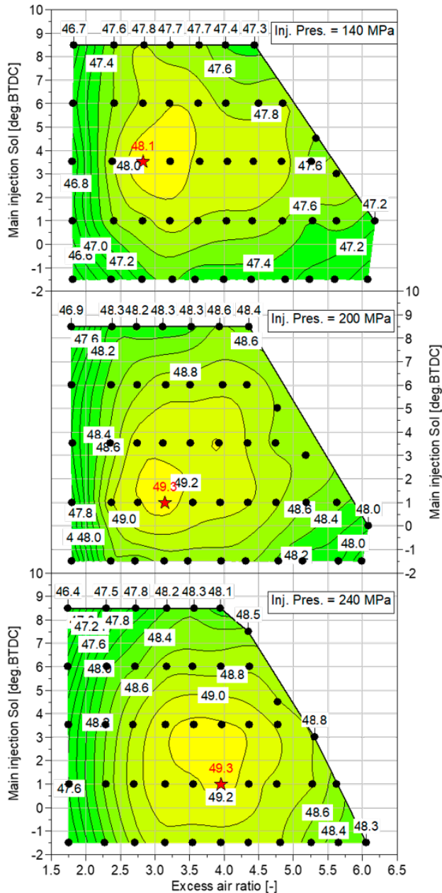
図2 燃料噴射量 66\text{mm}^3/\text{cycle} 、燃焼噴射圧力140MPa(上図)、200MPa(中図)、240MPa(下図)の条件での図示熱効率コンター図
