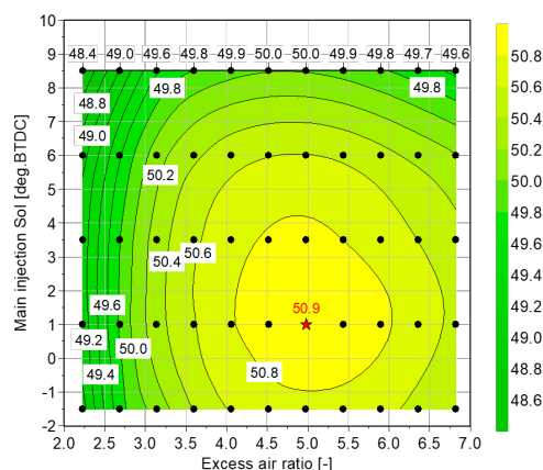
図1 燃料噴射圧力140MPa、噴射量66mm 3 /cycle条件下でのシミュレーションによる図示熱効率のコンター図
