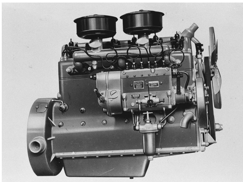
DA40型ディーゼルエンジン 水冷頭上弁(1939年ごろ)
