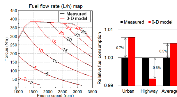
図2 シミュレーションの精度検証結果
