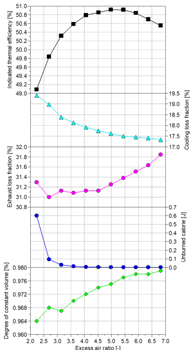
図8 HIDECSを用いた計算による(a)図示熱効率(b)冷却損失割合(c)排気損失割合(d)未燃熱量(e)燃焼等容度の比較
