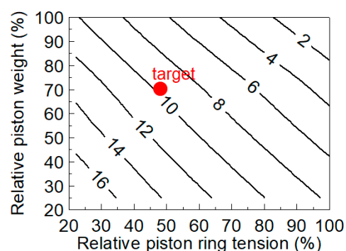
図12 ピストン重量とリング張力ピストン摩擦影響予測
