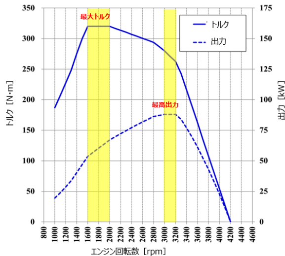
図5 RZ4Eエンジン出力・トルクカーブ
