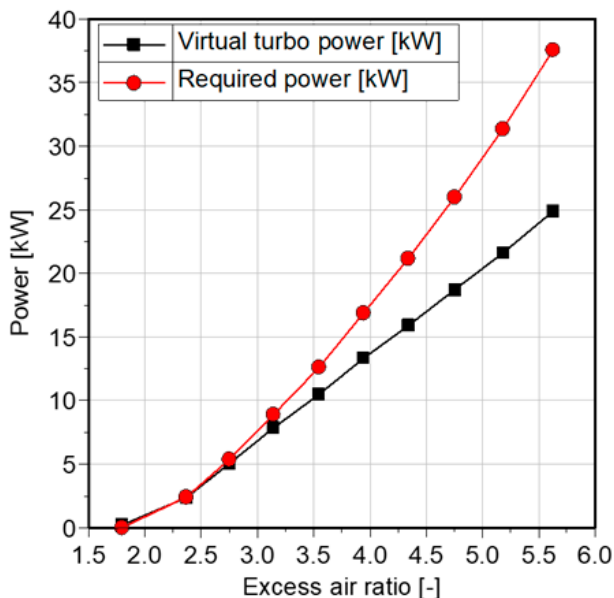
図12 各空気過剰率実現に必要なコンプレッサとタービンの仕事率の計算値比較
