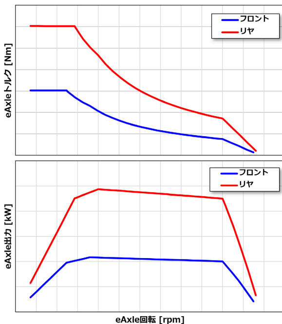
図3 フロントeAxle及びリアeAxle性能
