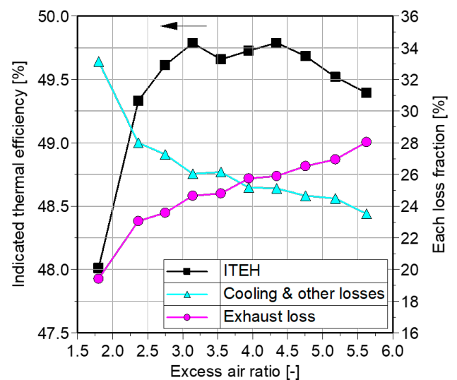
図4 燃料噴射量 66\text{mm}^3/\text{cycle} 、燃料噴射圧力200MPa、メイン噴射開始時期1.0deg.BTDCの条件での図示熱効率、排気損失及び冷却その他損失割合の比較
