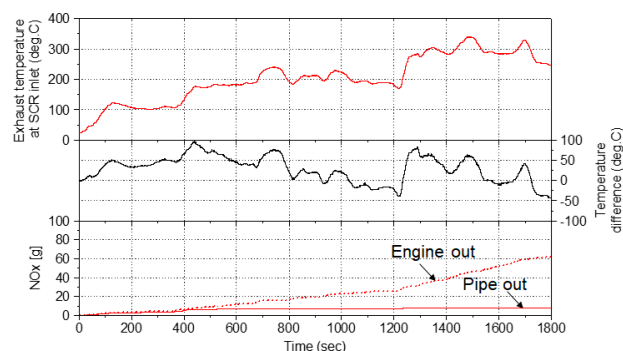
図15 WHTC冷間始動モード試験結果
