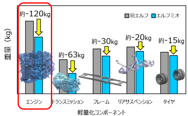
図15 各コンポーネントの軽量化
