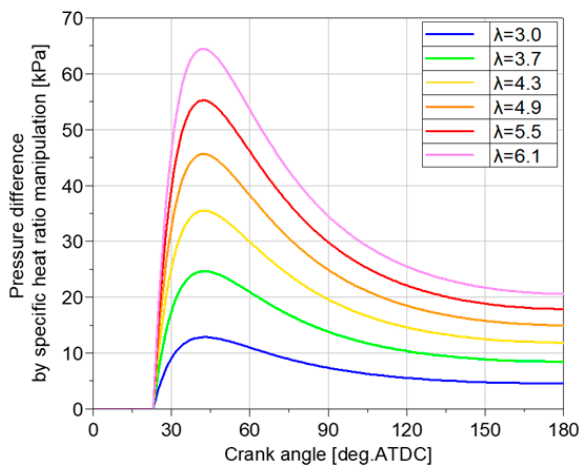
図10 HIDECSを用いた計算における空気過剰率の人為的な変更による圧力差の履歴の比較
