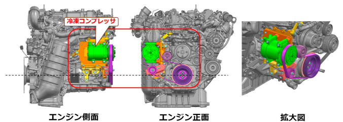
図17 冷凍バン架装仕様 エンジンレイアウト
