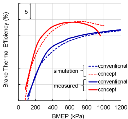
図17 正味熱効率の実機試験結果
