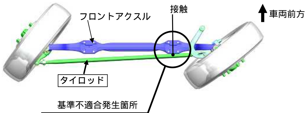
車両上方視
