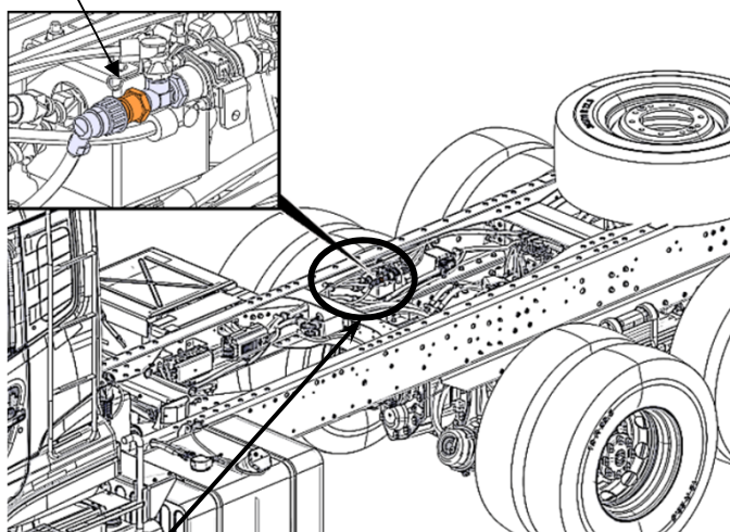
駐車ブレーキ用エアプレッシャーセンサ
