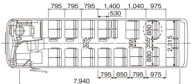
後部スライド2列サロン席 8列 スイング扉 カタログ番号【23】
