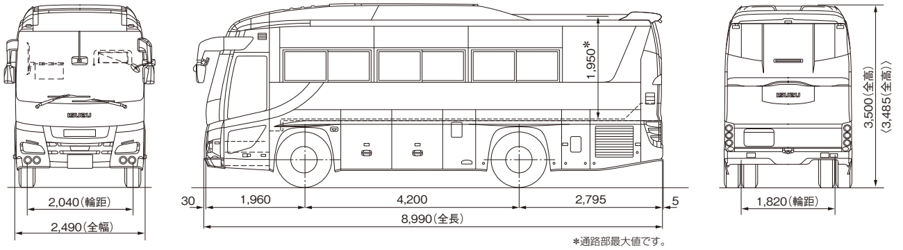
前向席 8列 スイング扉 カタログ番号【19】
