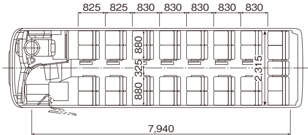
前向席 8列 スイング扉 カタログ番号【19】
