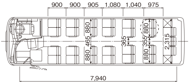
後部2列サロン席 7列 スイング扉 カタログ番号【22】
