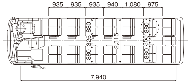
後部1列サロン席 7列 スイング扉 カタログ番号【20】
