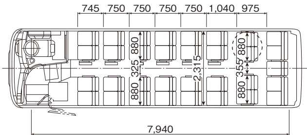
後部1列サロン席 8列 スイング扉 カタログ番号【21】
