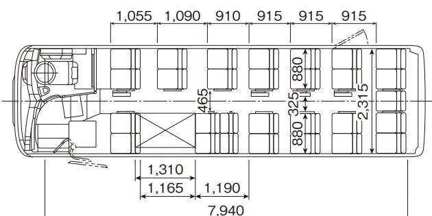
リフト付(ホイールベース間) 7列 スイング扉 カタログ番号【24】
