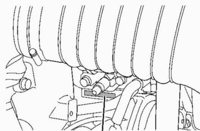
エンジン番号打刻位置
