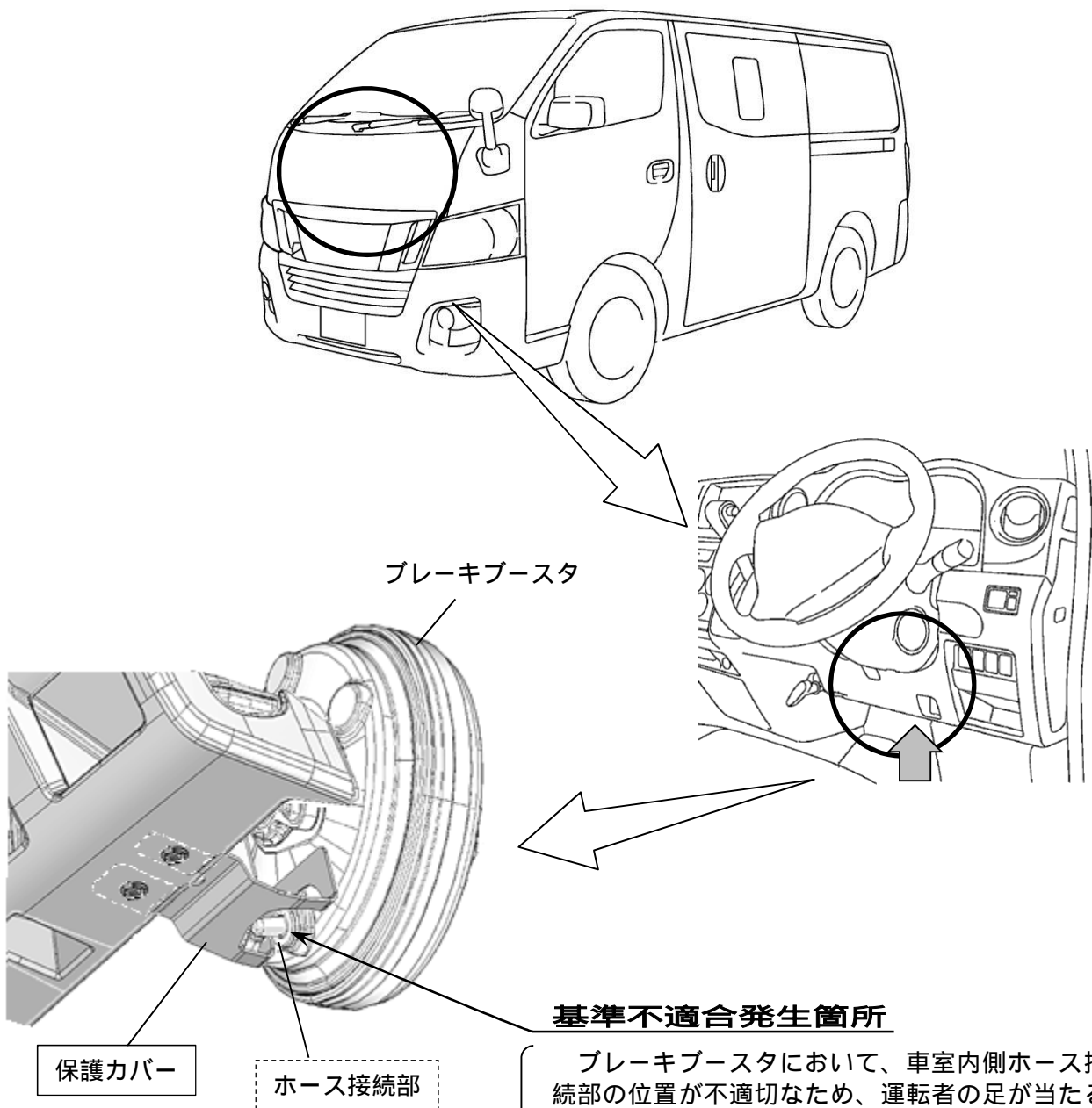
矢視図
